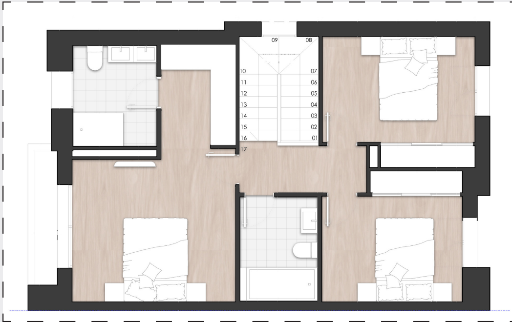
PLANTA PRIMERA
