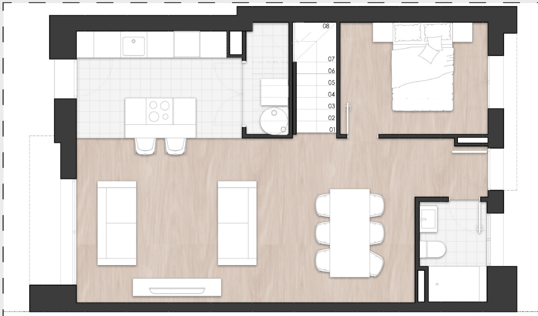
PLANTA BAJA
