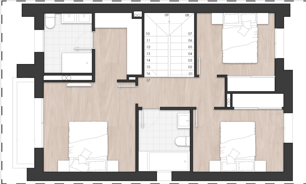
PLANTA PRIMERA
